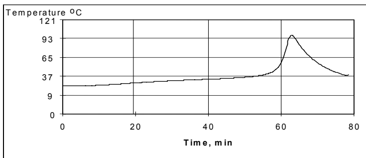
Typische Reaktivitätskurve Für at 23°C (10 grams) 5
