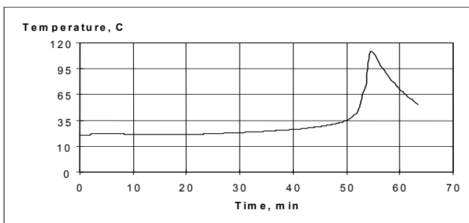
Typische Reaktivitätskurve für at 23°C (10 grams) 5
