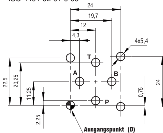
ISO 4401-02-01-0-05
