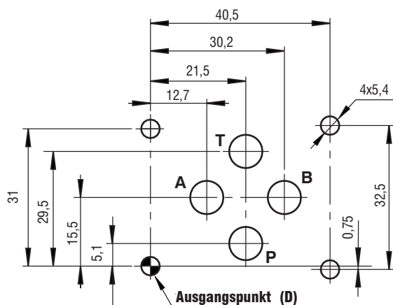
ISO 4401-03-03-0-05
