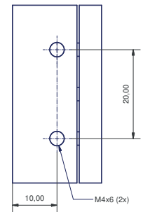
Halteblock LED-Kopf
